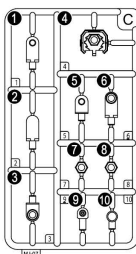
パーツC×4 (スチロール樹脂:PS)
