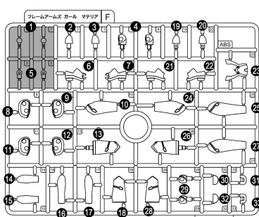
パーツF (ABS樹脂: ABS)
