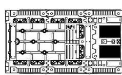
ベース2 (ABS樹脂：ABS)
