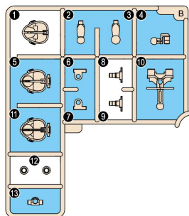
パーツB (ABS)
