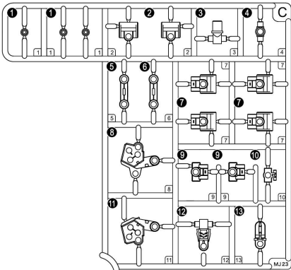
パーツC×2 (スチロール樹脂:PS)
