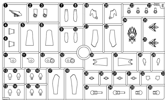
パーツE (ABS)
