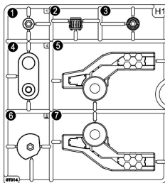
パーツH1 (スチロール樹脂:PS)
